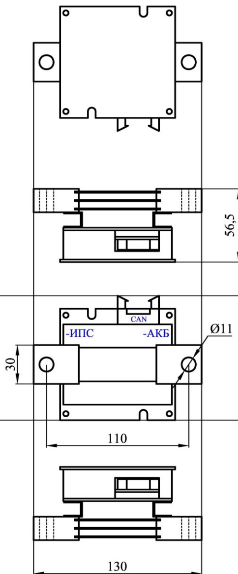
МОДУЛЬ ИЗМЕРЕНИЯ ТОКА АКБ 300А (НА БАЗЕ 75ШСММ3-300А)
